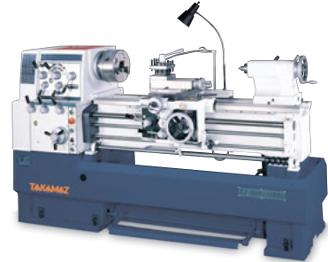
ECOCA (台湾) 汎用旋盤 SJ460×1000G
